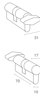
Cilindro llave-llave o llave-mariposa
